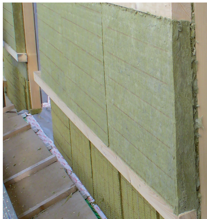
Abb. 6: Befestigung durch Klemmen
